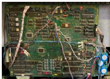
プリント板
