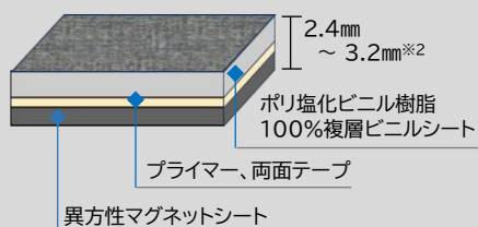
【シートの断面図】
